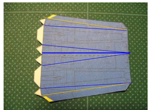
21. 機体下部を付ける Glue the Body under side together.
