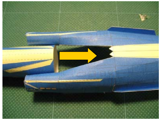
⑪. 機体上部 Body upside1.
