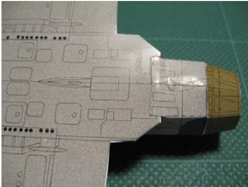
27. J:カナード右を組み立てる。 Fold and glue the J.Canard Right.
