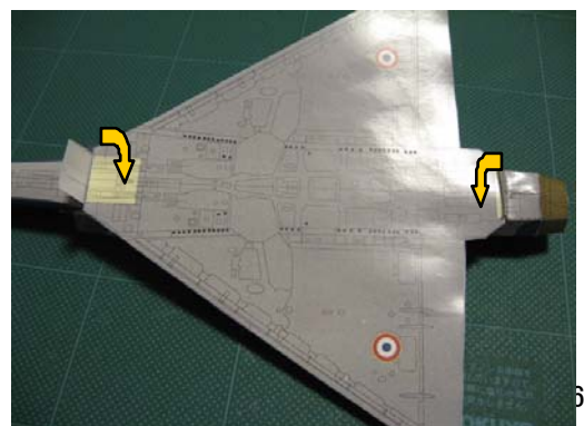
24 機体と主翼を糊付ける。(下側) Glue together main wing and body. (underside)
