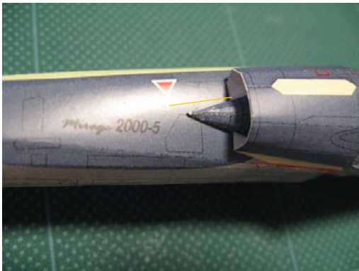
23 機体と主翼を糊付ける。 Glue together main wing and body.
