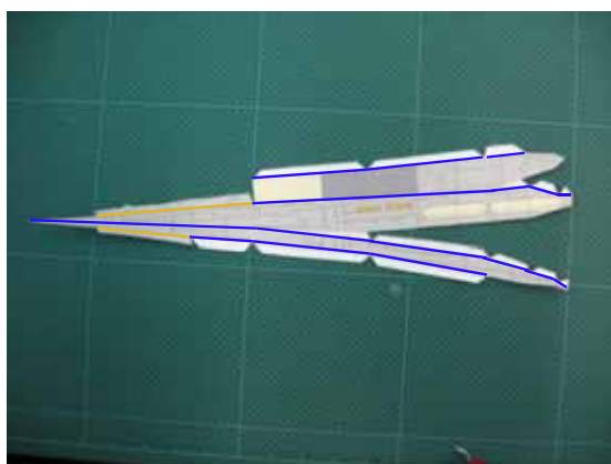
3 7 . J,K : エンジン脇の折り方
