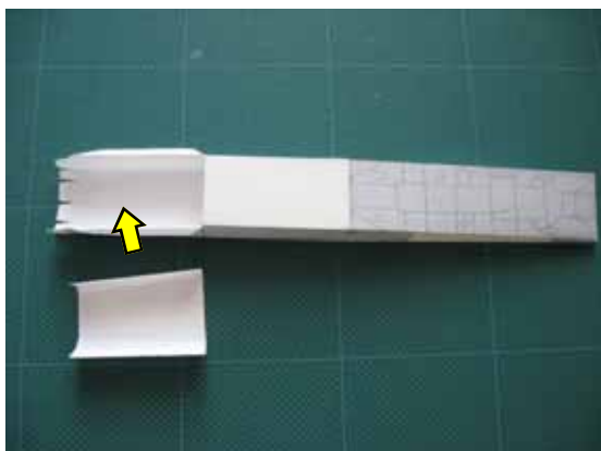
21 . 機体下部を主翼に取り付ける
