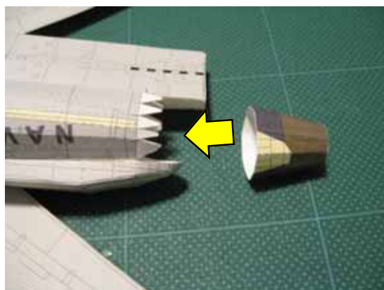
46 . エンジン
